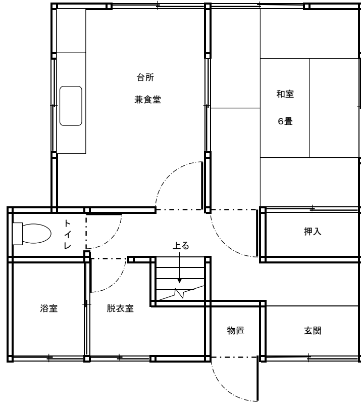
1階
