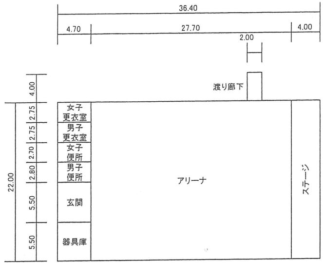
③ 1階
