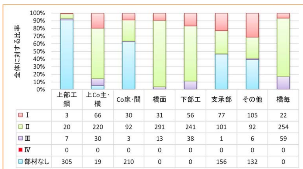
図 1.2.2 全管理橋梁の損傷傾向図
