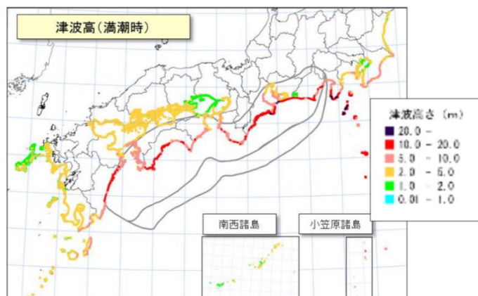
【「駿河湾～紀伊半島沖」に「大すべり域+超大すべり」域を設定した場合の津波高分布図】
