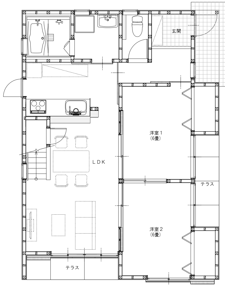
1階平面図
